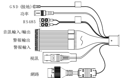
圖 1-2 纜線 II
