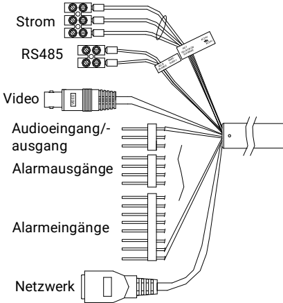
Abbildung 1-1 Verkabelung I
