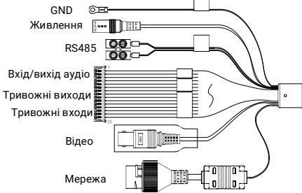
Рисунок 1-2. Кабелі II
