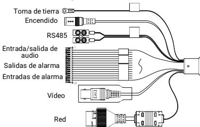
Imagen 1-2 Cables II
