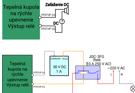
Obrázok 1-2 Káble II
