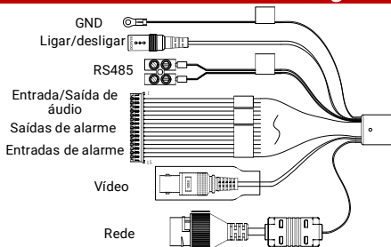
Figura 1-2 Cabos II
