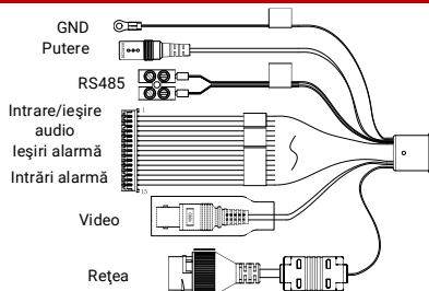
Figura 1-2 Cabluri II
