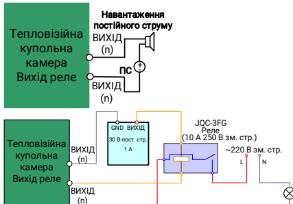
Рисунок 1-2. Кабелі II
