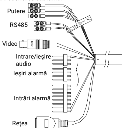
Figura 1-1 Cabluri I
