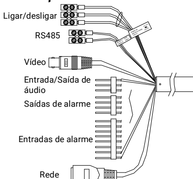
Figura 1-1 Cabos I
