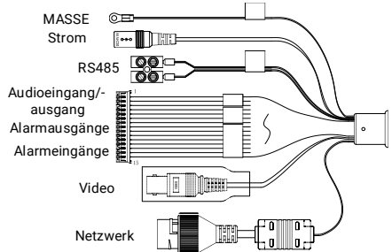
Abbildung 1-2 Verkabelung II
