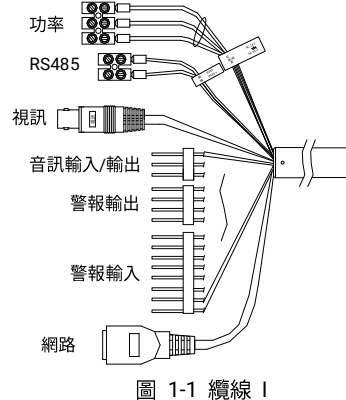
圖 1-1 纜線 I
