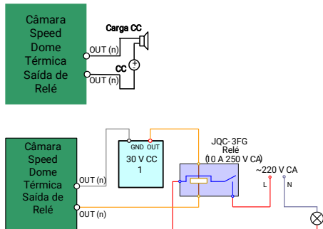
Figura 1-2 Cabos II
