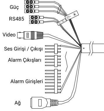
Şekil 1-1 Kablolar I
